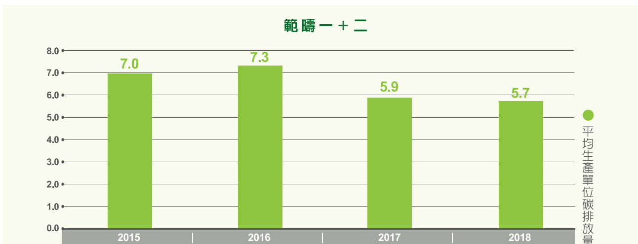
研華台北廠區及辦公室 2015 年 ~ 2018 年度範疇一與範疇二溫室氣體平均每生產單位排放量 (單位為公斤 CO 2 e/ 年) 圖 4.13
